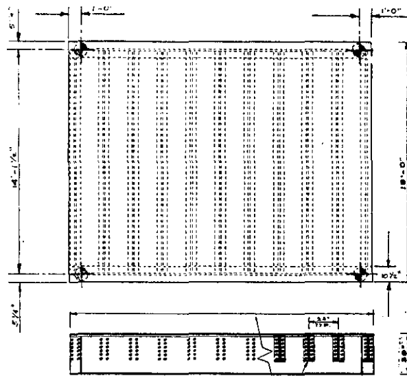
Weighbridge/Châssis récepteur
