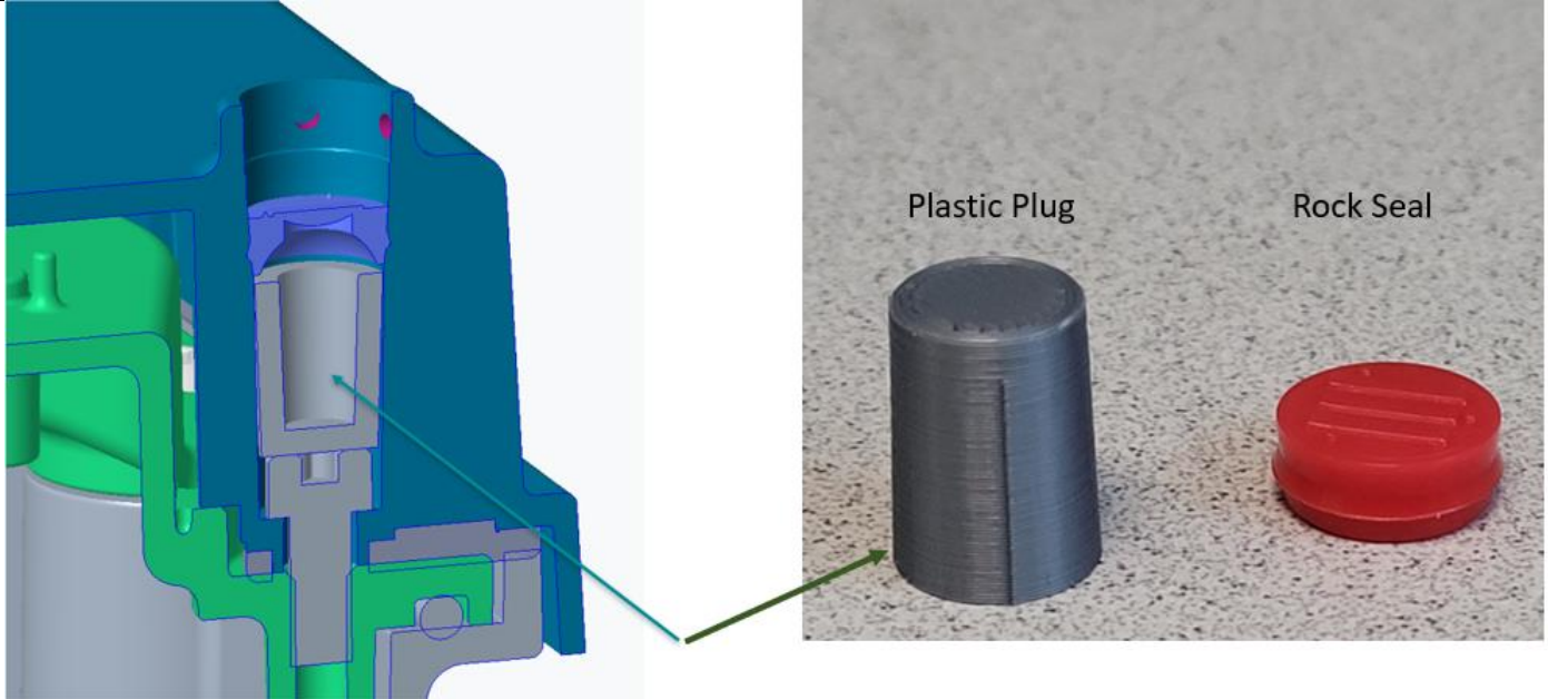
Figure 6: Position of the plastic plug above the screw head inside the screw hole / Position du bouchon en plastique au-dessus de la tête de la vis à l'intérieur du trou de la vis
