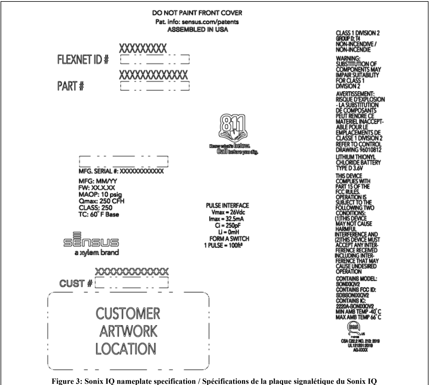
Figure 3: Sonix IQ nameplate specification / Spécifications de la plaque signalétique du Sonix IQ
