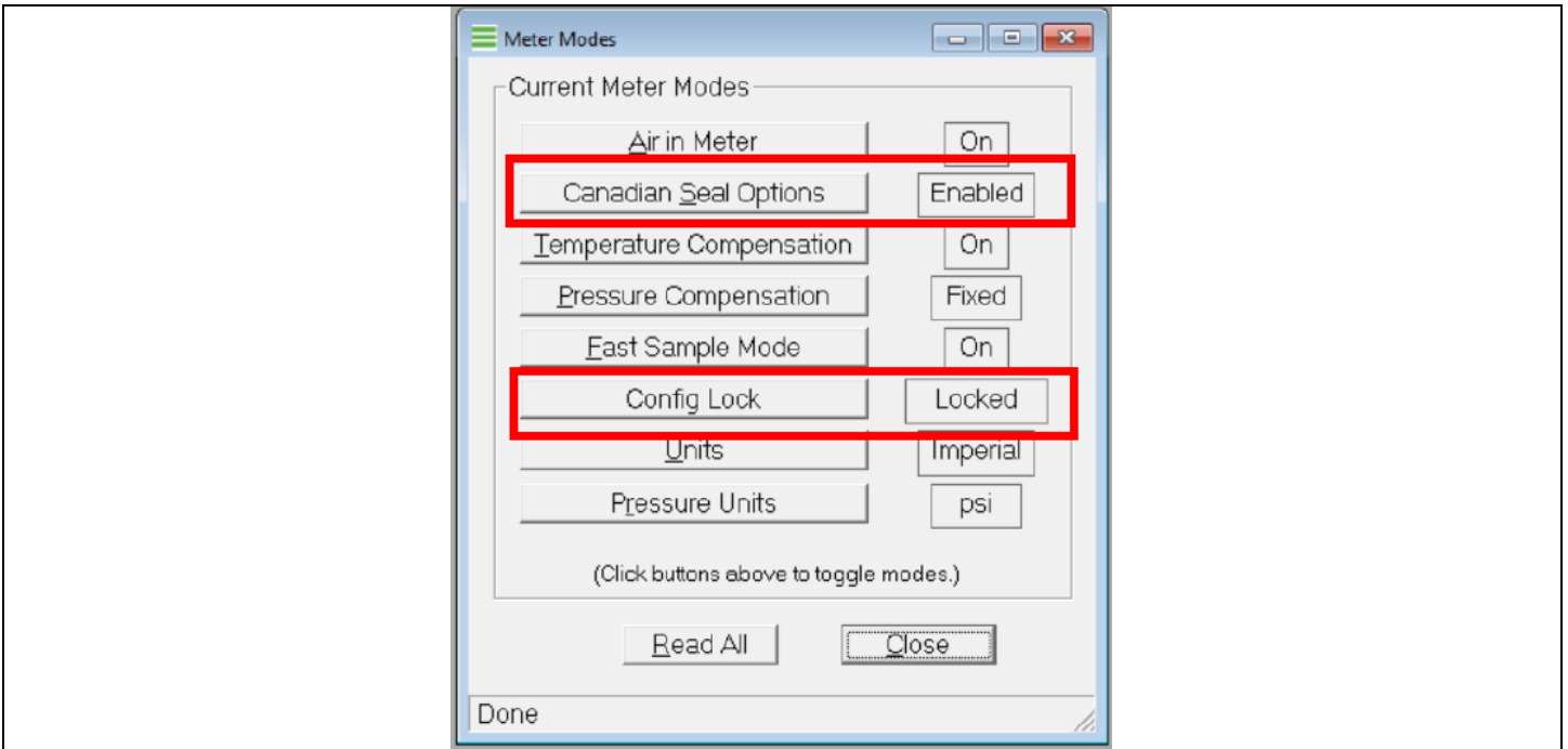
Figure 8: Using SonixCom, Canadian Seal is enabled with the Config Lock 'locked' / Avec SonixCom, le sceau canadien est activé avec le verrou de configuration "verrouillé".
