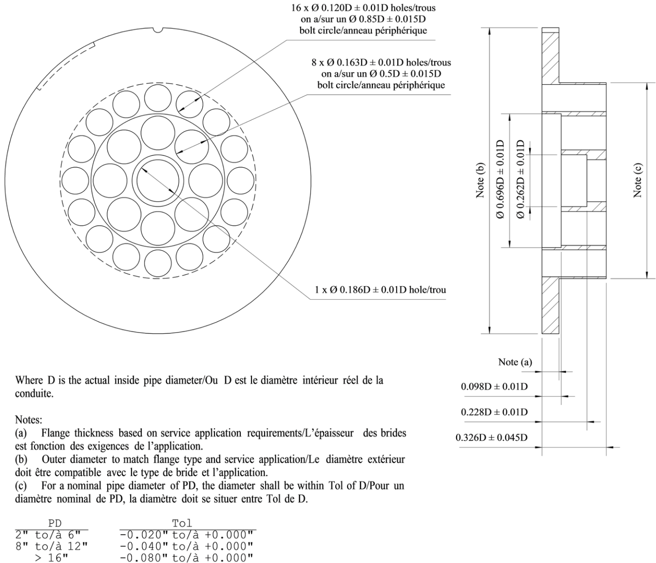
Figure 1. CPA 55E Flow Conditioner \ Tranquilliseur d'écoulement CPA 55E
