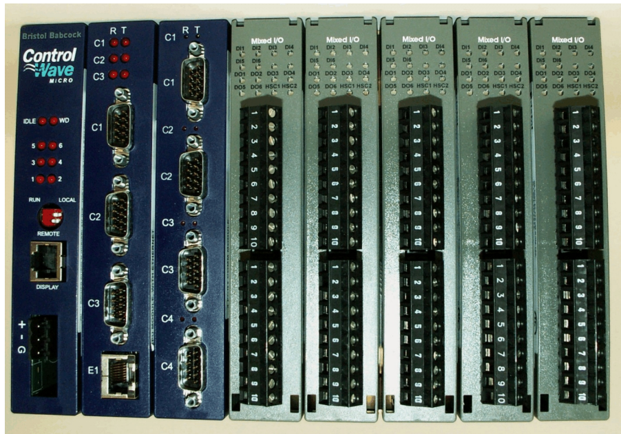
Figure 1 Base chassis populated with from left to right: a power supply, a CPU, a communications and five I/O modules / Châssis de base doté, de gauche à droite : d'un module d'alimentation en énergie, d'un module UCT, d'un module de communication et de cinq modules E/S
