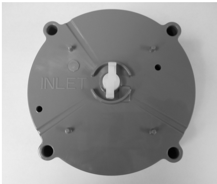
Figure 12: 100G ERT, Part No. ERG-5000-007 (Rear View) / N° de pièce ERG-5000-007 (vue arrière)
