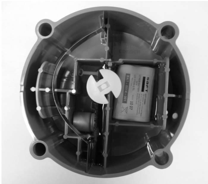
Figure 11: 100G ERT, Part No. ERG-5000-007 (Front View) / N° de pièce ERG-5000-007 (vue de face)
