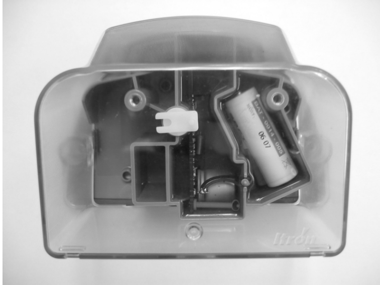
Figure 3 : 100G ERT, Part No. ERG-5000-005 (Front View) / N° de pièce ERG-5000-005 (vue de face)
