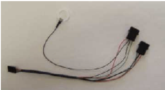
Figure 4. Ground strap connected to the electronics ground via the battery cable assembly / Tresse de mise à la masse connectée à la masse des circuits électroniques via le cablage de la batterie
