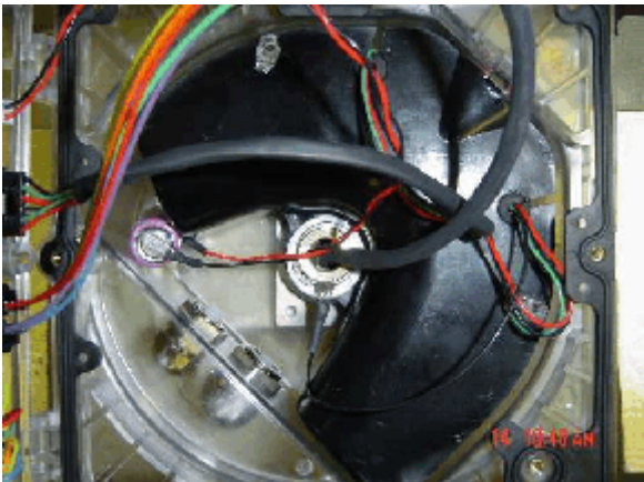
Figure 5. Ground wire attached to center of housing/Fil de mise à la masse fixé au centre du boîtier
