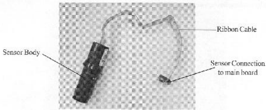
Figure 4 : Type 1 REI Rotary Sensor / Capteur rotatif REI de type 1
