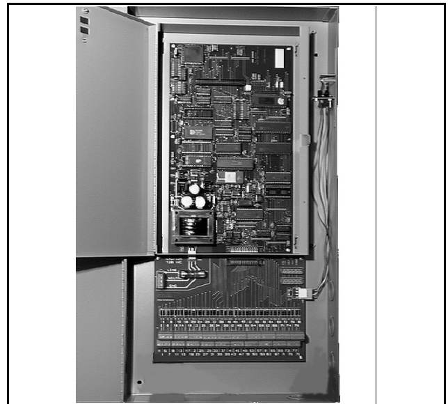
Rev. 5, EMP-II – New Layout, Doors open (with T2 card) Rév. 5, MSÉ-II – Nouvelle configuration, portes ouvertes (avec la carte T2)
