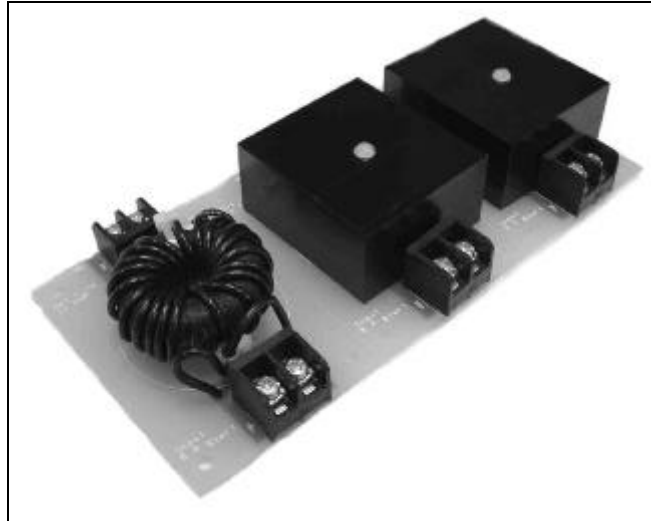
Interposing Transducer PCB, Old layout Carte de circuits imprimés « Interposing Transducer », ancienne configuration
