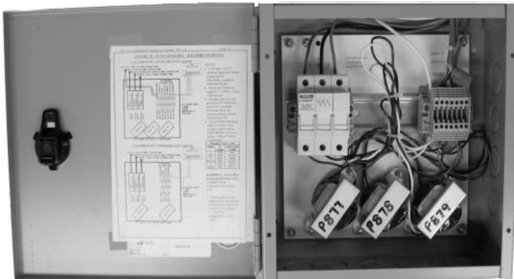
Voltage (Potential) Transformers/Transformateurs de tension
