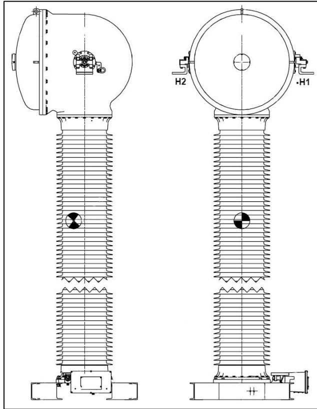
Current transformer / Transformateur de courant
