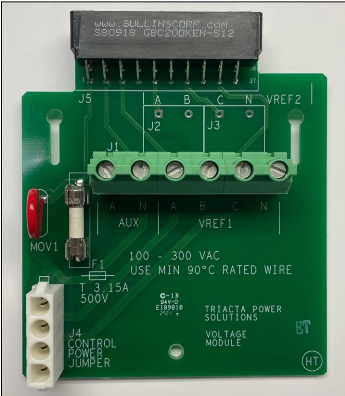
Single reference voltage / Tension de référence singulaire
