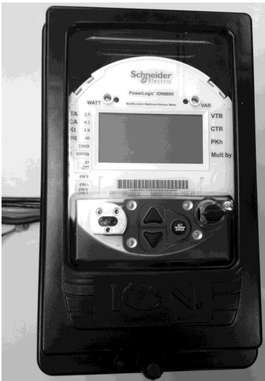
Switchboard type meter. / Compteur pour tableau de distribution.
