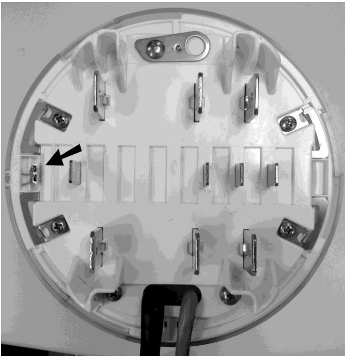
Single seal on a socket type meter / Sceau unique sur un compteur de type socle.
