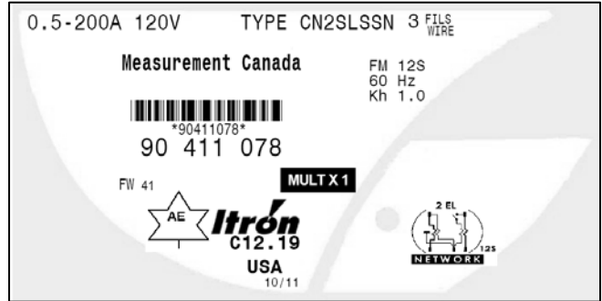
Nameplate for CENTRON II C12.19 / Plaque Signalétique pour le CENTRON II C12.19
