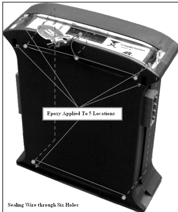
Sealing and epoxy locations of the TX-2005A meter / Scellage et emplacements d'époxy du TX-2005A
