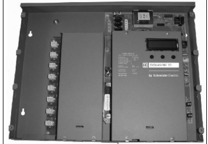
PowerLogic E4805 Meter / Compteur PowerLogic E4805
