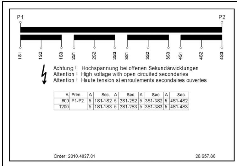
Schematic/Schéma
