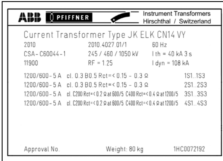
Nameplate/Plaque signalétique
