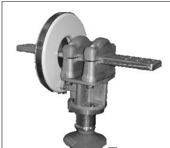
Optical sensor head/Tête de détection optique
