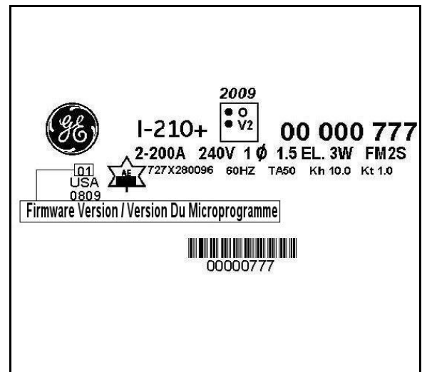
Nameplate With Firmware Version / Plaque signalétique avec version du micrologiciel
