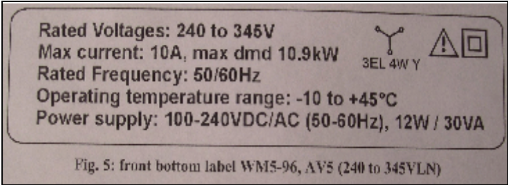
Front Bottom nameplate / Plaque signalétique du bas-avant
