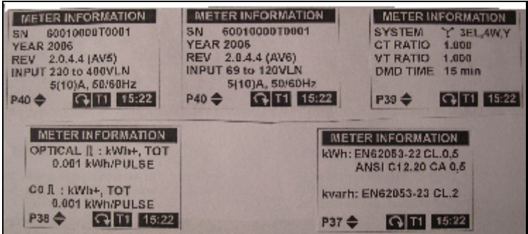
Nameplate Information In the Display / Information de plaque signalétique dans l'afficheur
