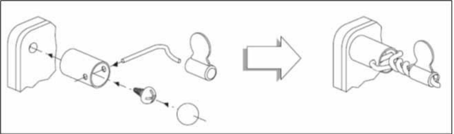
Ball and Can Hardware Kit / Trousse de matériel balle boîte
