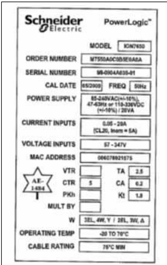
Auxiliary Nameplate / Plaque signalétique supplémentaire
