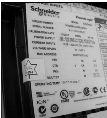
Tamper Evident Nameplate / Plaque signalétique inaltérable PARTIE 5 – Plaques Signalétiques et Photo
