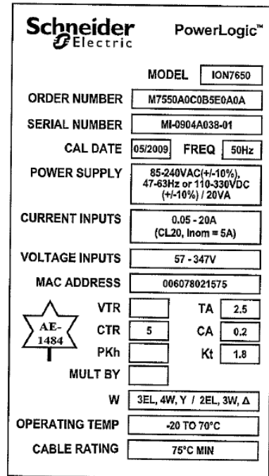
Auxiliary Nameplate / Plaque signalétique supplémentaire
