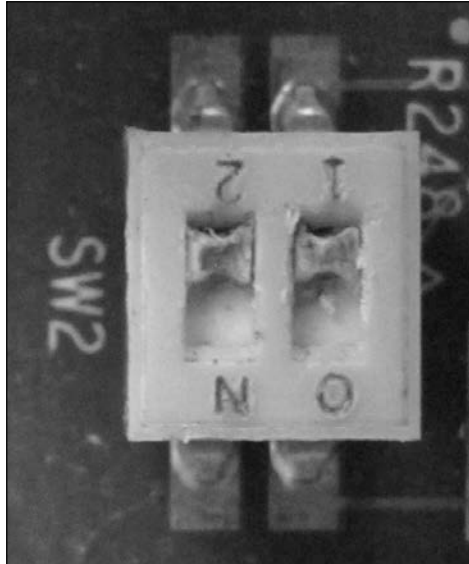
SW2 programming switch in 1-2 position / L'interrupteur de programmation SW2 en position 1-2
