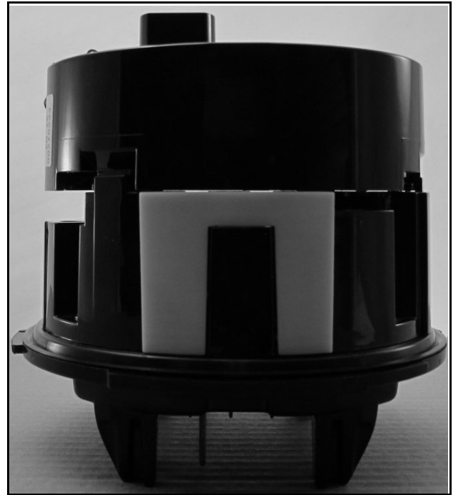
Polycarbonate insert (shown in white, production version is black) in inner housing/ Pièce en polycarbonate (en blanc dans la photo, la version de production est noire) insérée dans la coque intérieure
