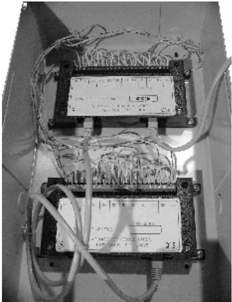
Pulse Input Board / Carte d'entrée d'impulsions d'impulsions
