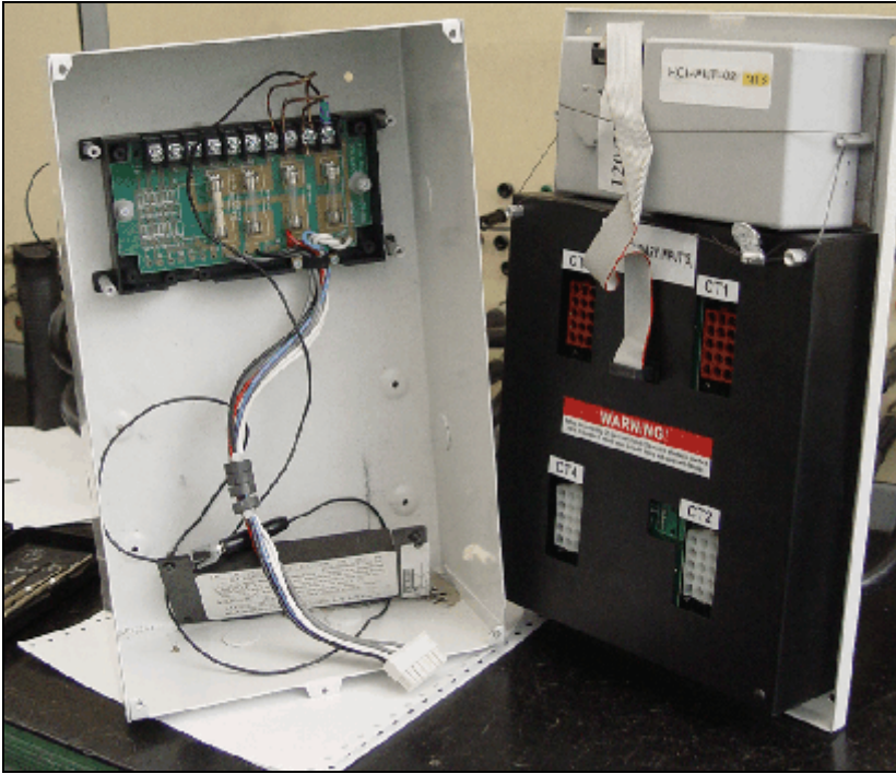
Head unit with PT input board / Unité Principal et carte d'entrée des TP
