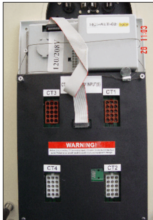
Sealed head unit with CT inputs / Scelage de l'unité principale et entrée des TC
