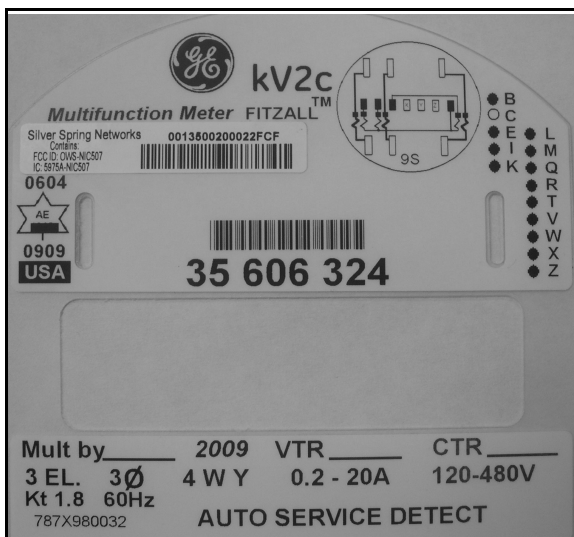
kv2c markings with new SSN module / Marquages de kv2c avec le nouveau module SSN
