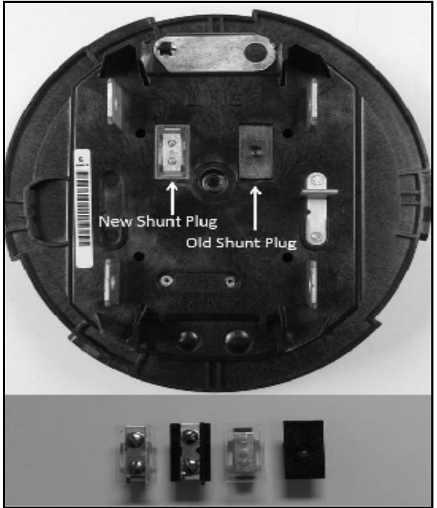
New Centron Shunt Plug / Nouveau bouchon shunt de Centron
