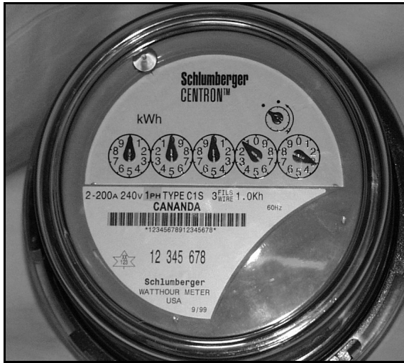
C1S Clock Dial *1 / Mimutrie à tambours *1
