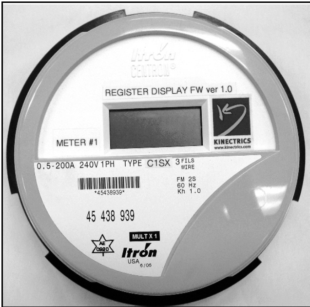
C1SX with Kinectrics / CiSX avec Kinectrics
