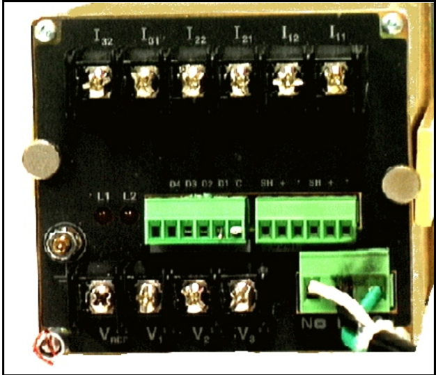
Rear Face of 7300 ION Meter / Face arrière du compteur 7300 ION
